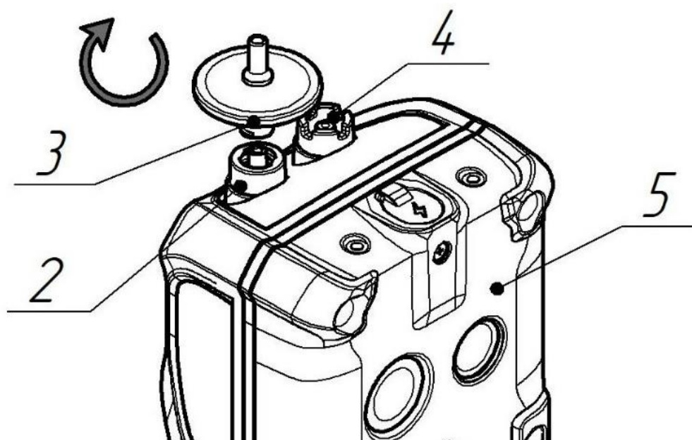
Рисунок 12 – Фильтр на насосном модуле
