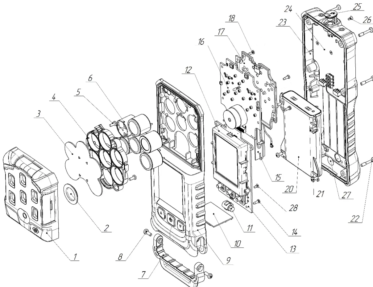
Рисунок 13 – Внешний вид газоанализатора в разобранном состоянии
