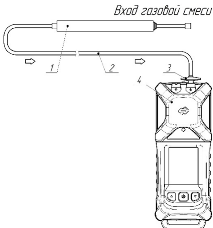
Рисунок 4 – Соединение насосного модуля с зондом
