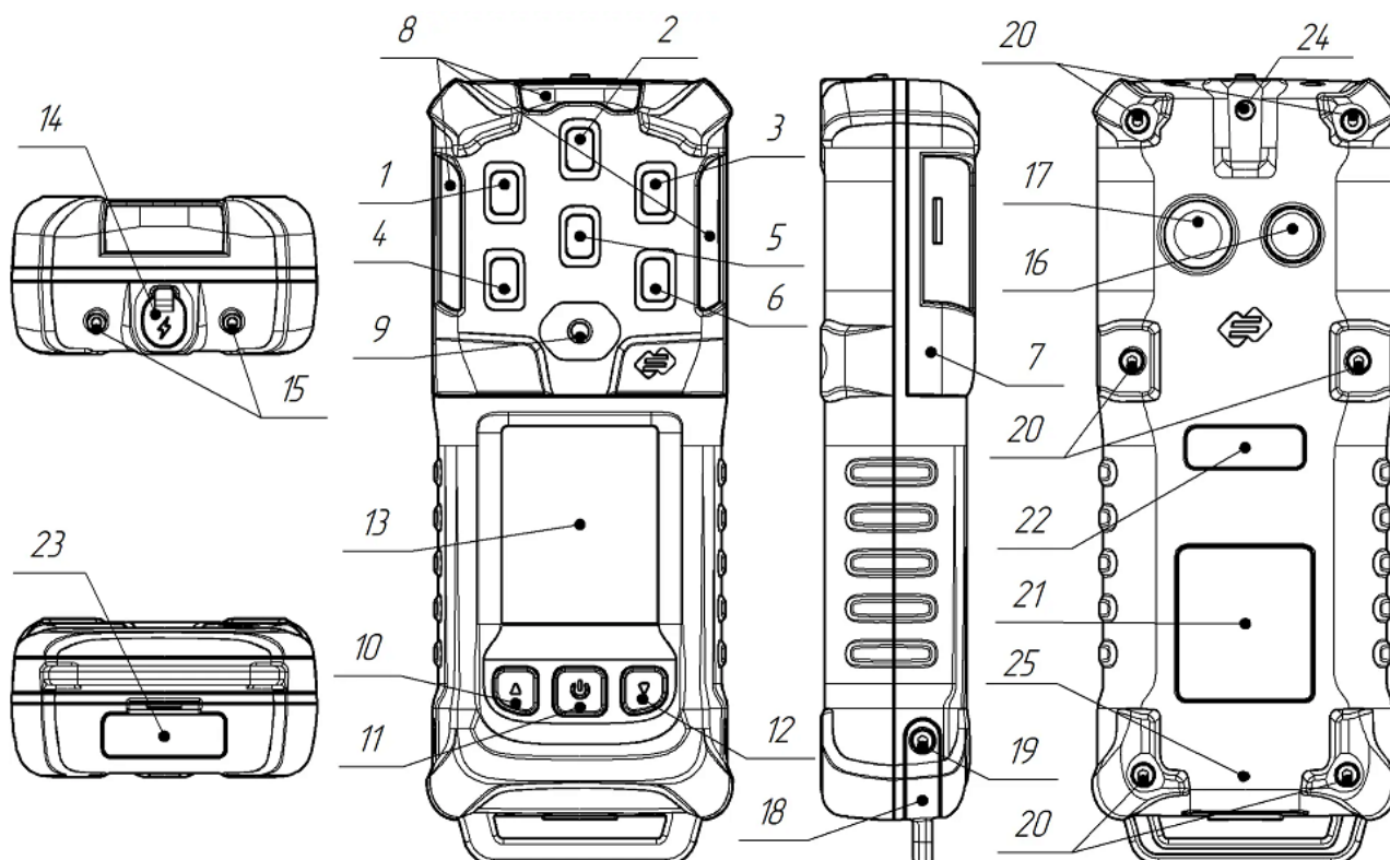
Рисунок 1 – Внешний вид газоанализатора в сборе
