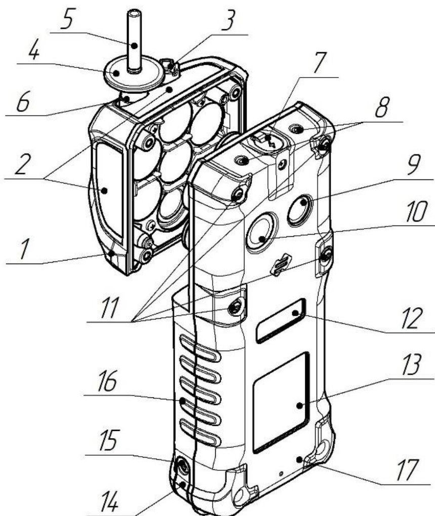
Рисунок 3 – Присоединение насосного модуля к газоанализатору
