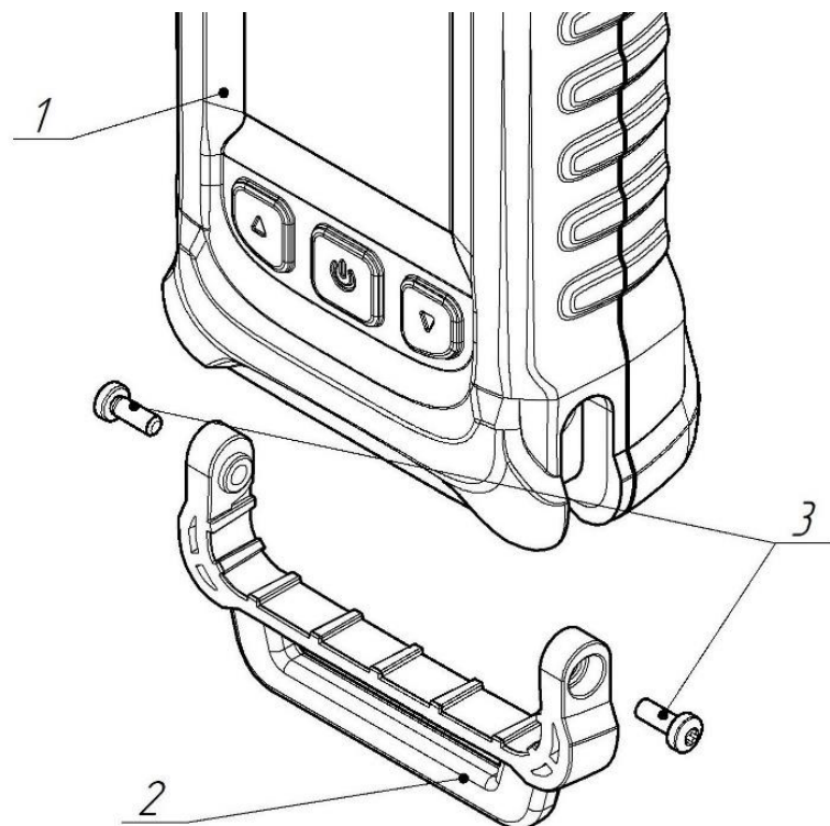
Рисунок 16 – Внешний вид процедуры замены держателя ремня
