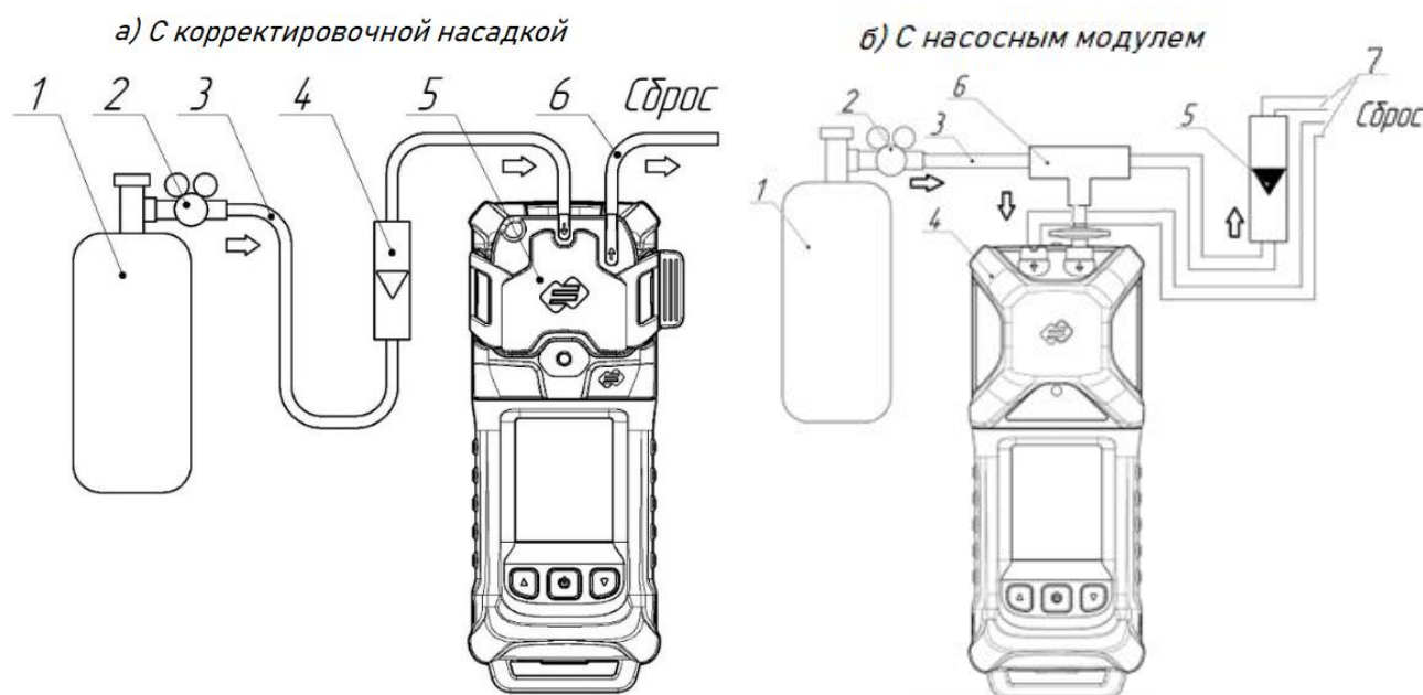
Рисунок 7 – Схема соединений для корректировки газоанализатора
