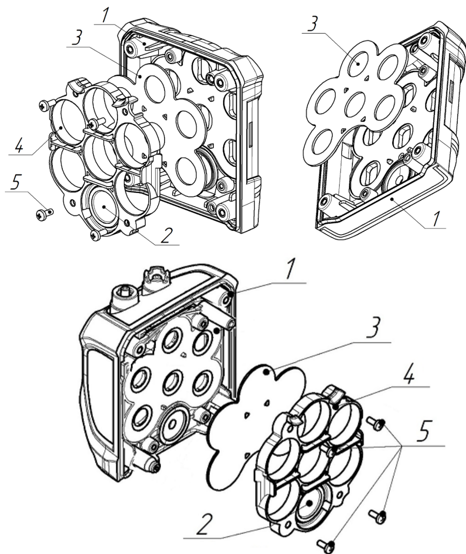
Рисунок 10 – Внешний вид крышки сенсоров в разобранном состоянии
