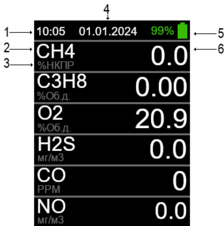
Рисунок 5 – TFT-дисплей газоанализатора
